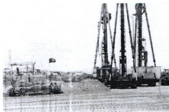
Thi công cọc cát đường cao tốc Hà Nội - Thái Nguyên
